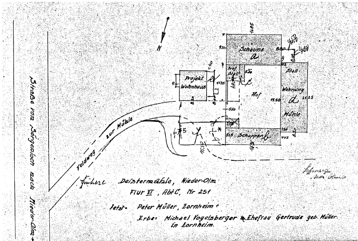
Lageplan zum Neubau eines Wohnhauses an der Mittleren Ecklocher Mühle in den 1930er Jahren. 45
